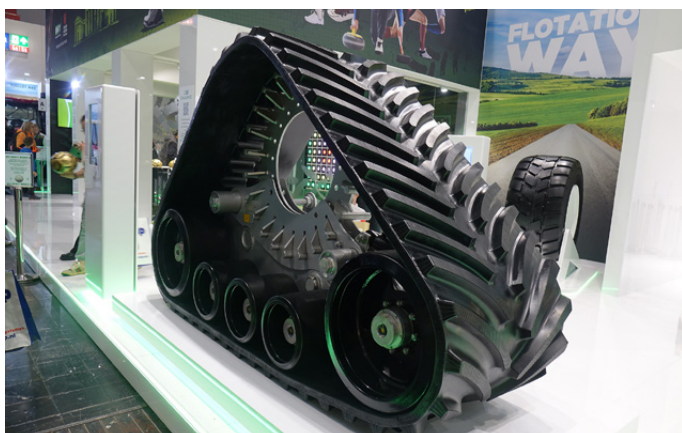
Il cingolo BK T71 nella misura 34" x 6" x 44
